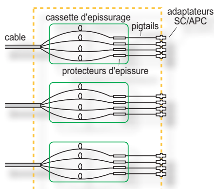
Diagramme de montage de FKH-312.
